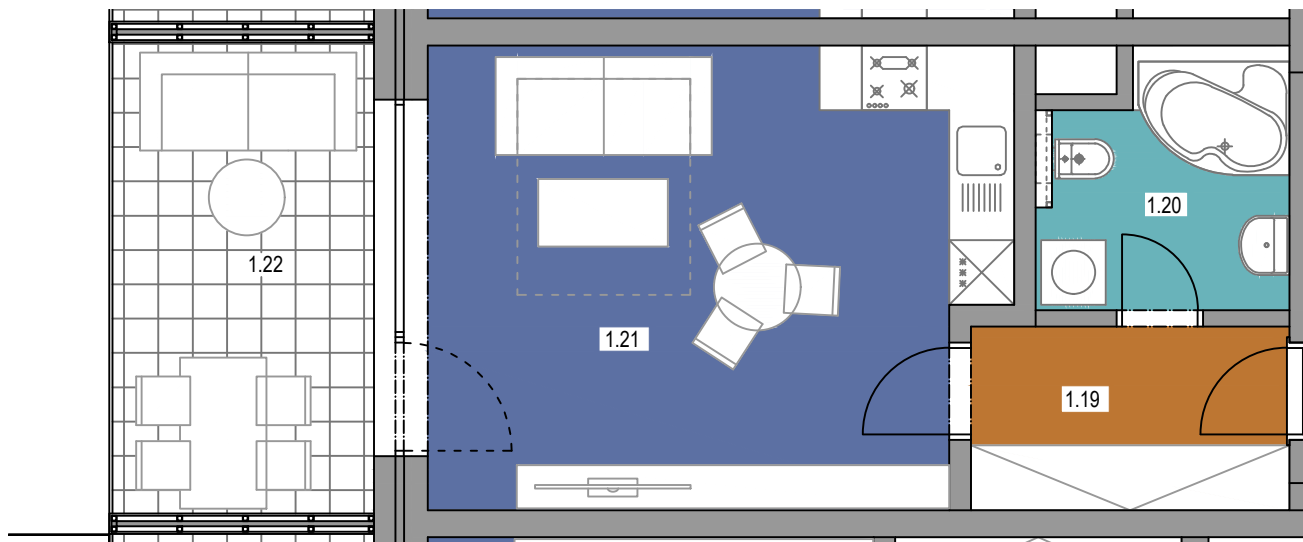
PŮDORYS 1.NP
